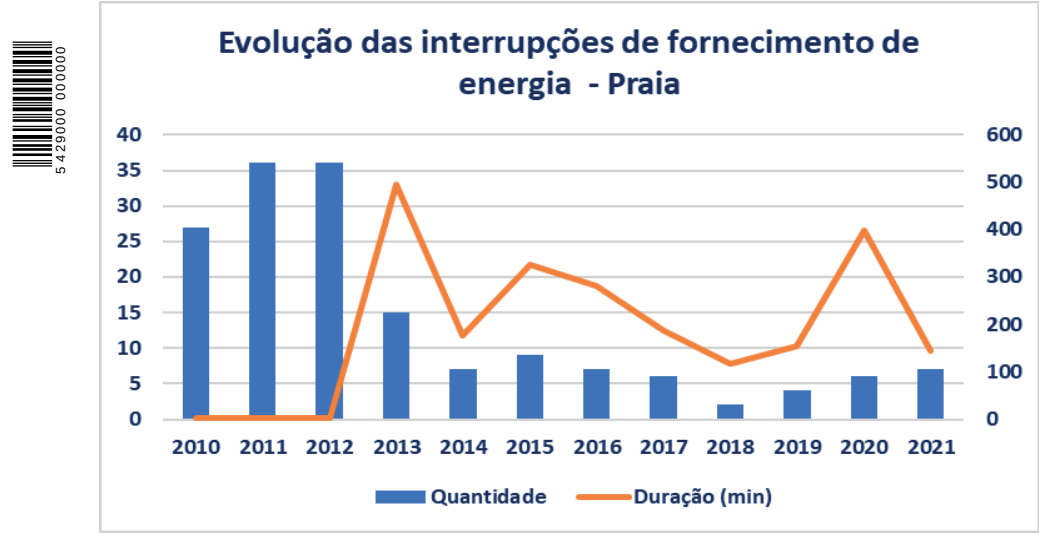
Figura 21 – Evolução das interrupções de fornecimento de energia elétrica na rede da Praia (Fonte: Relatórios anuais da ELECTRA ( www.electra.cv ))
