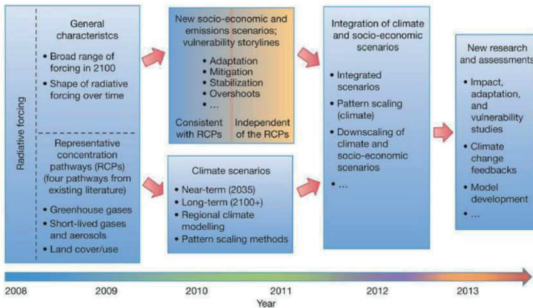
Figura 27: Desenvolvimento paralelo de cenários climáticos e cenários de emissões socioeconômicos do RCP (Fonte: Moss et al., 2010).
